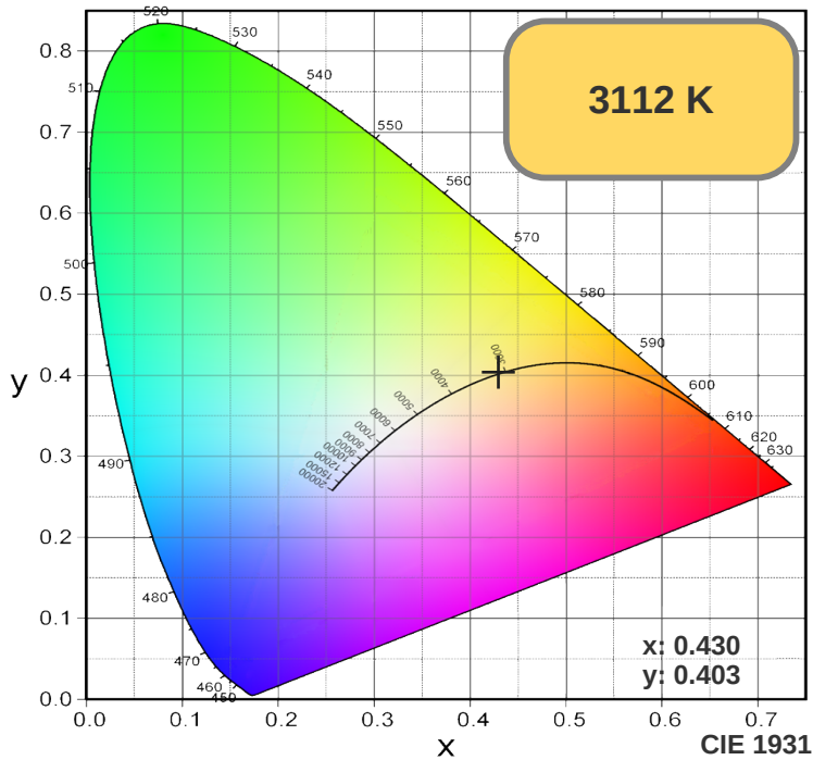
TM30: 84.5
