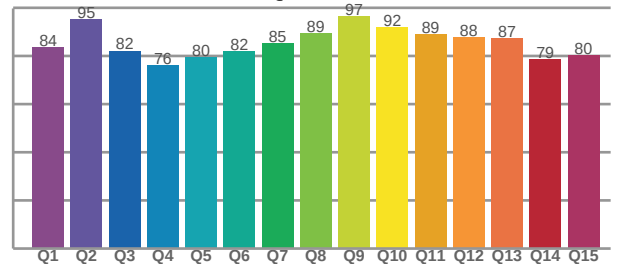
CQS: 84.4
