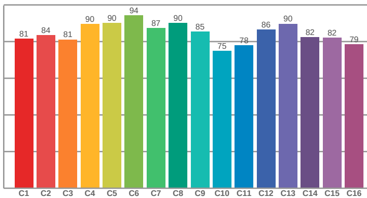
TM30: 84.5
